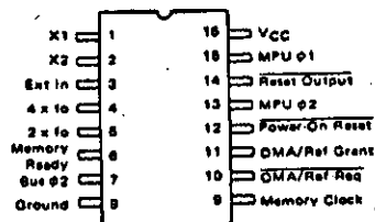
Slika 1. Razporeditev nožic za taktni generator MC6875
